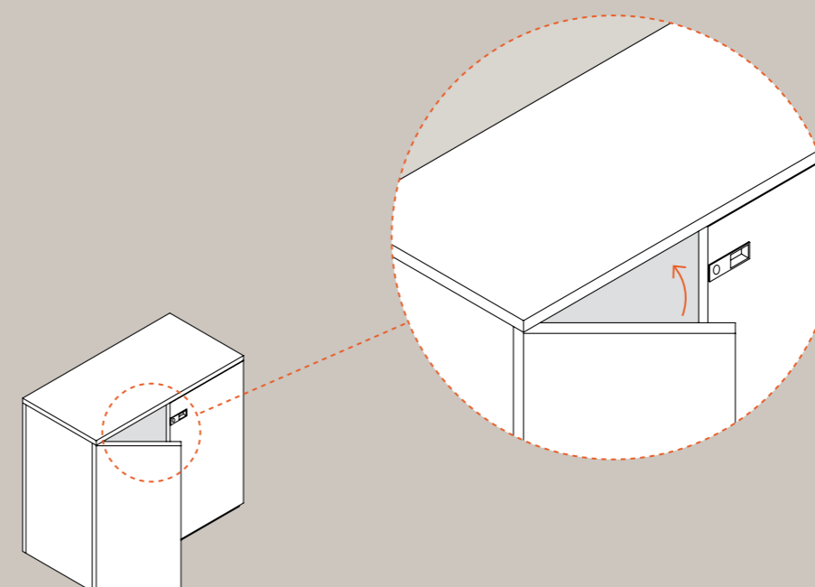
les charnières sont amorties et se referment automatiquement au-delà de 30°
